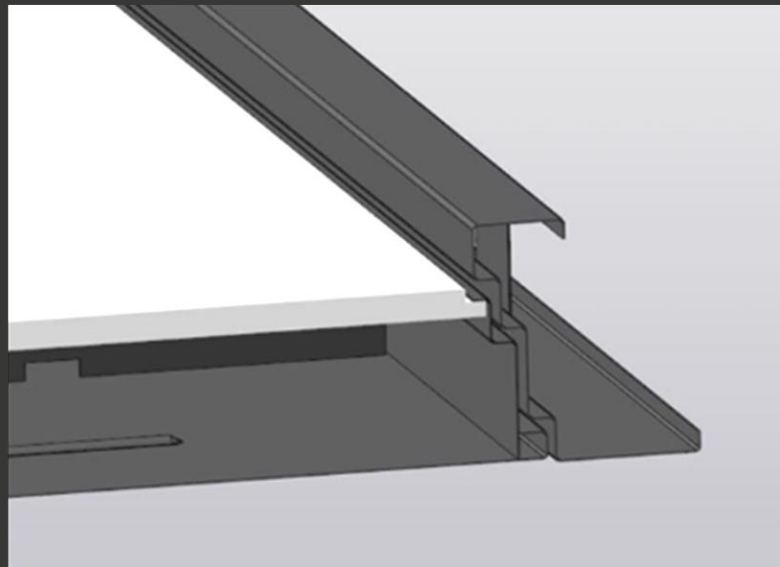
Три контура уплотнения
